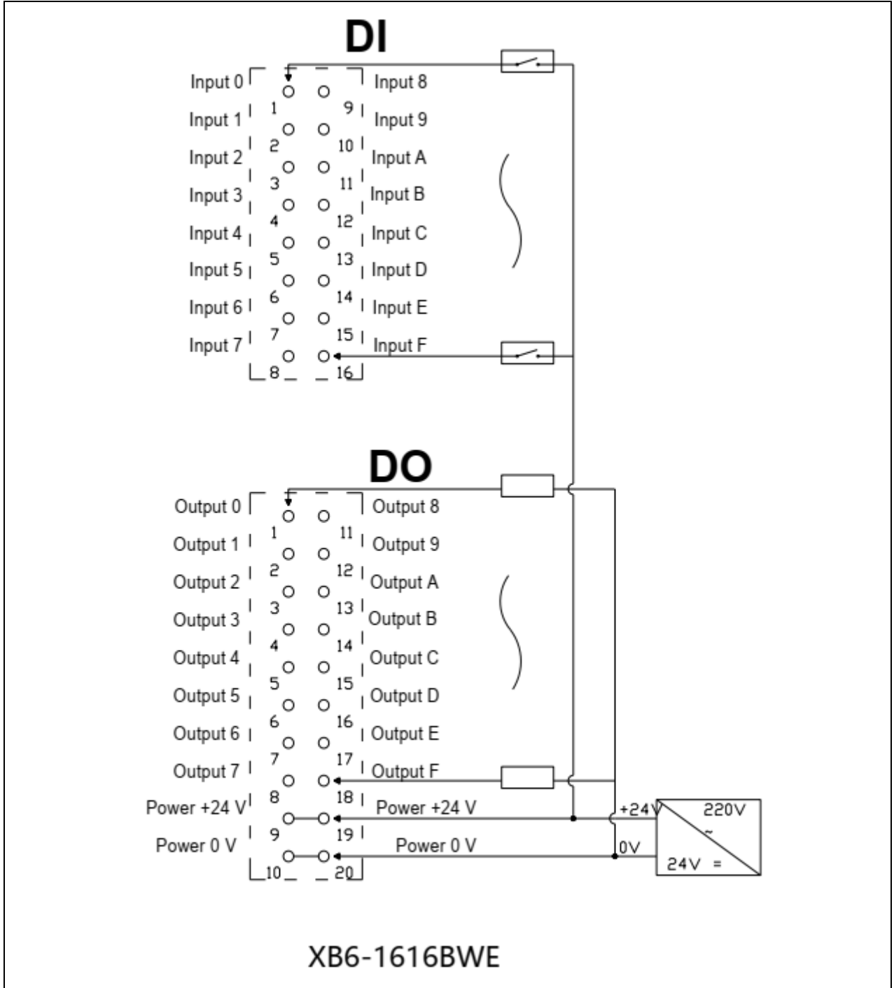
图 11.1 输入输出模块接线图 (XB6-1616BWE)
