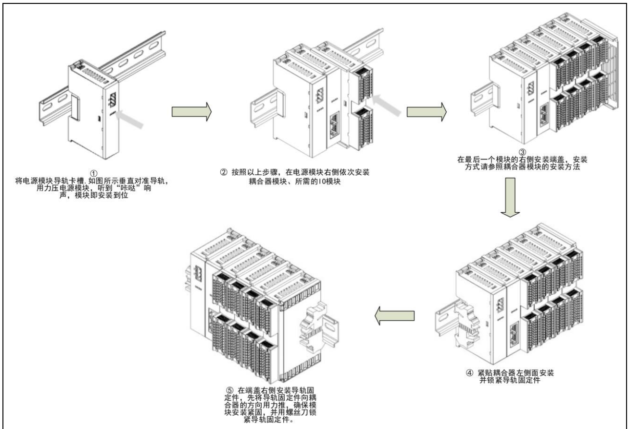
图 6.1 模块的安装示意图 (XB6-1616BWE)
