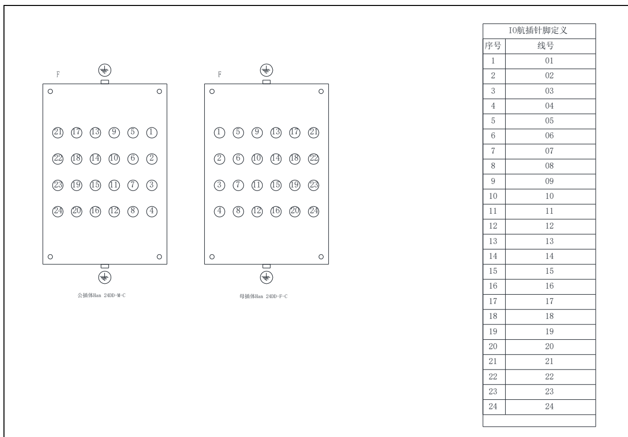
图 11.17 IO 航插接线图
