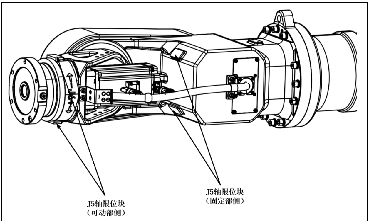
图 3.16 J5 轴机械式制动器位置 (ER100B-3000, ER100B-3500-DW, ER130B-3200)
