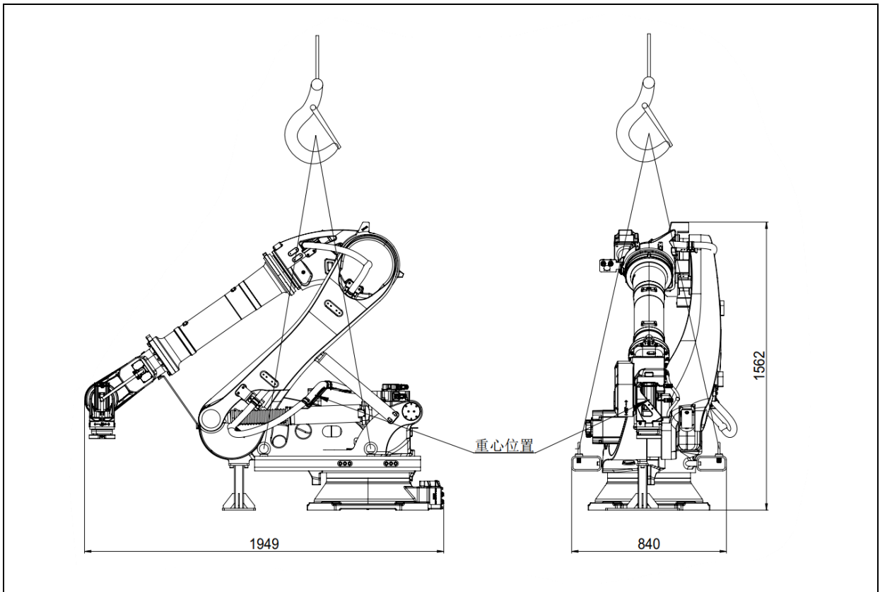
图 1.10 机器人起重机搬运示意图 (ER100B-3500-DW)
