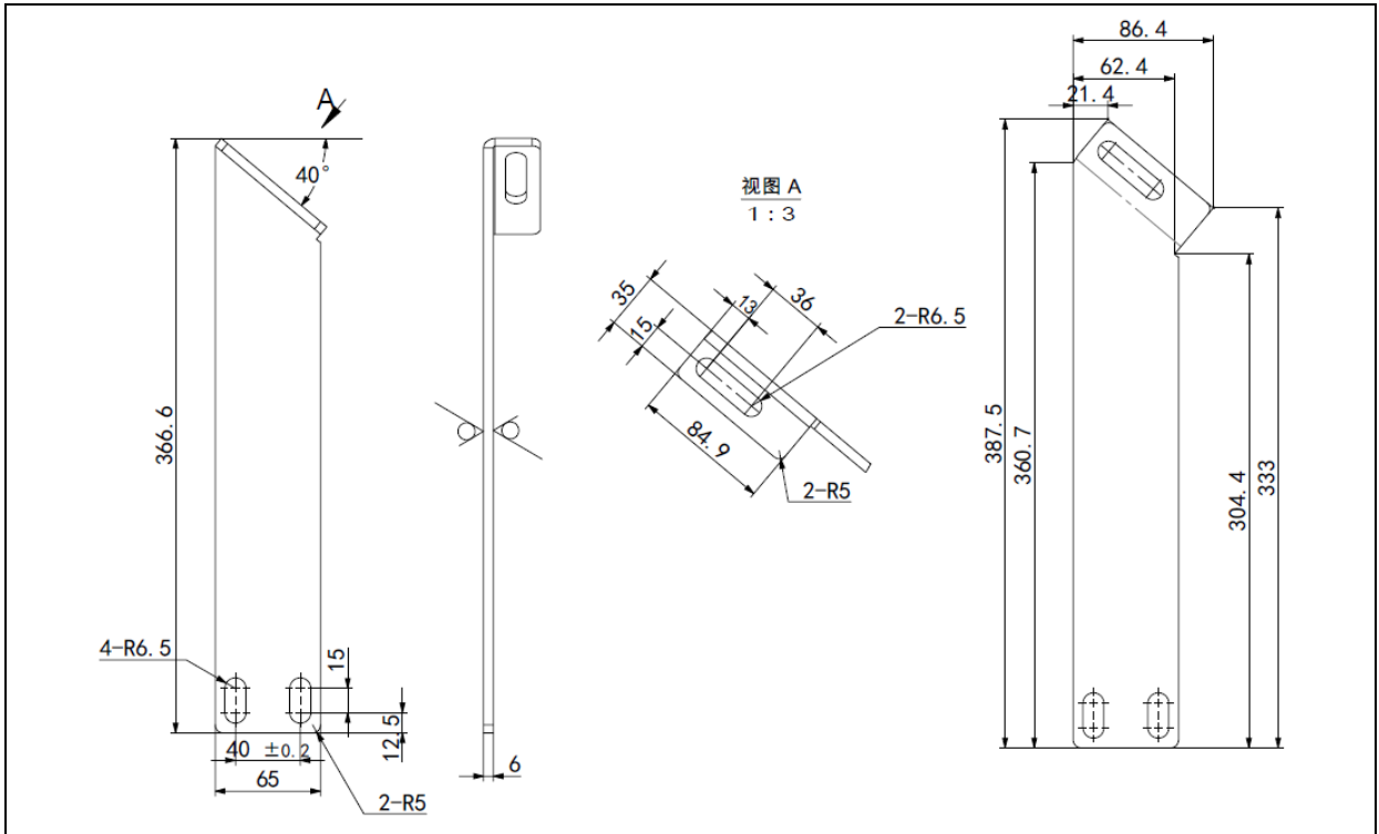
图 1.1 机器人固定支架示意图 1 (ER100B-3000,ER130B-3200,ER170B-2650,ER220B-2650)
