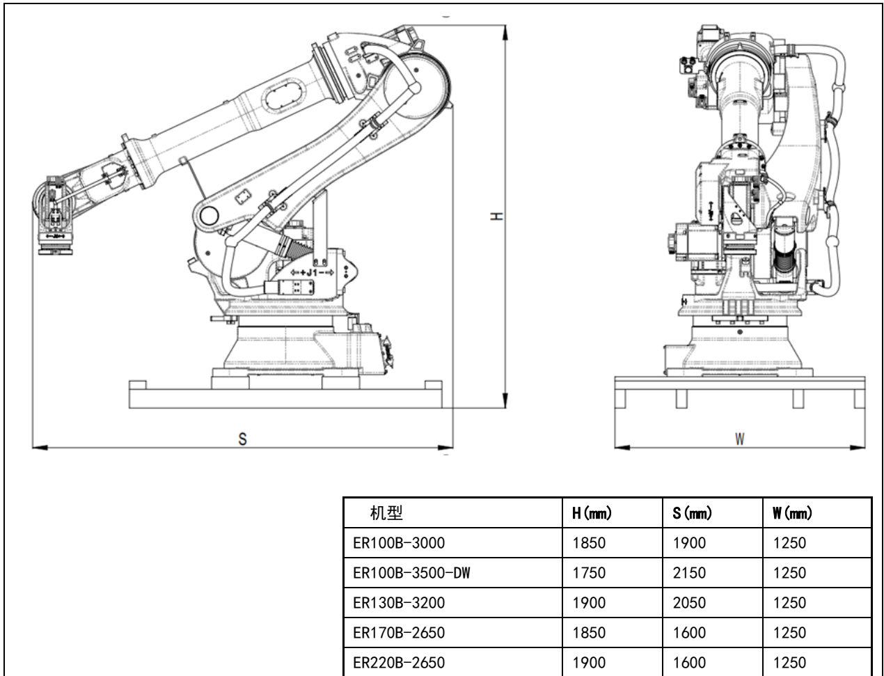
图 1.11 机器人存储空间尺寸图
