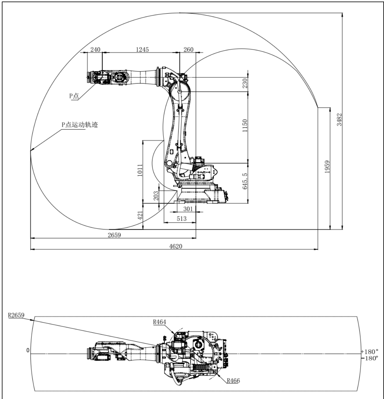
图 3.9 动作范围图 (ER220B-2650)
