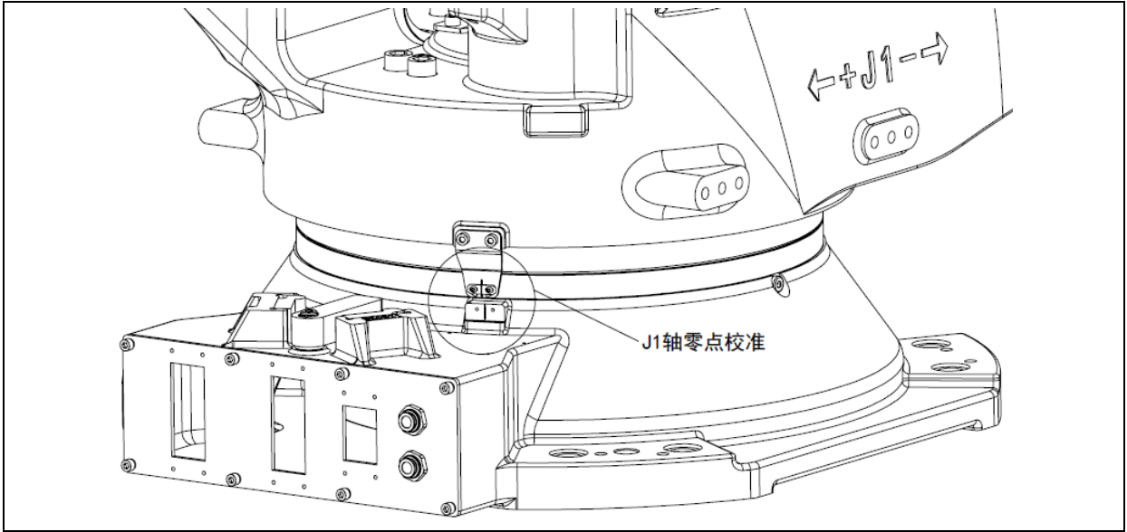
图 6.4 J1 轴零点校准示意图 (ER100B-3500-DW)
