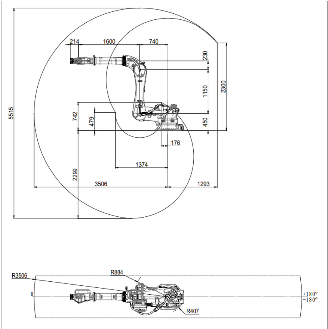
图 3.6 动作范围图 (ER100B-3500-DW)
