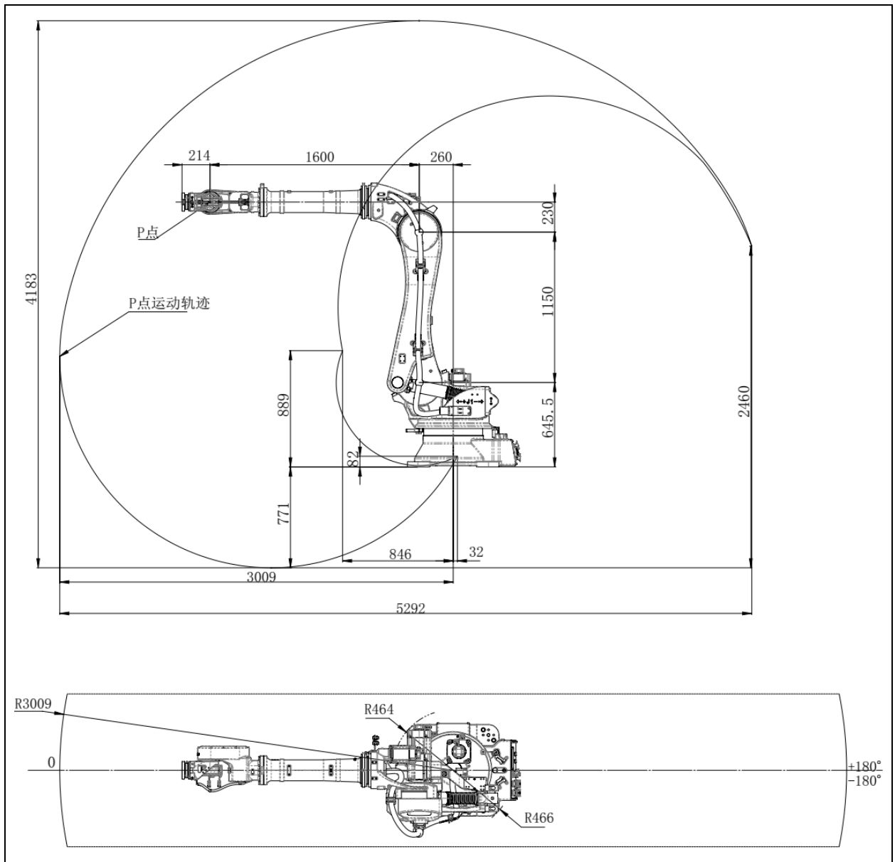
图 3.5 动作范围图 (ER100B-3000)
