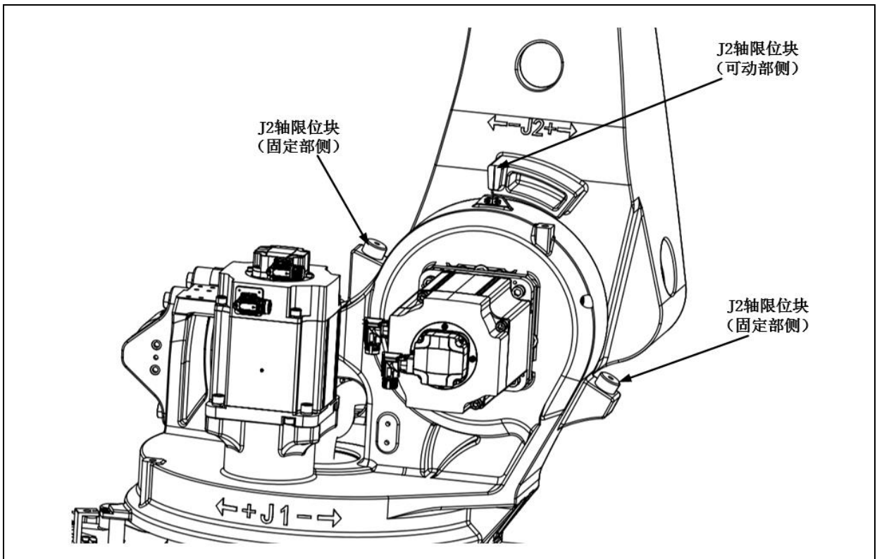
图 3.13 J2 轴机械式制动器位置 (ER100B-3000, ER130B-3200, ER170B-2650, ER220B-2650)
