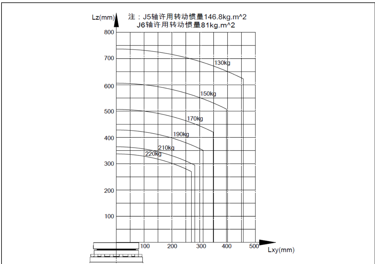
图 3.21 手腕部负载条件 (ER220B-2650)
