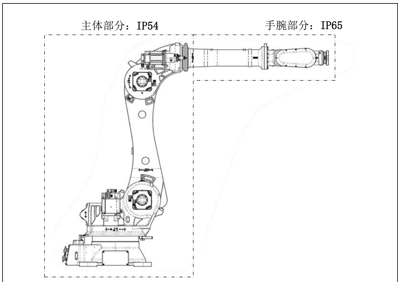
图 1.17 机器人防护等级示意图
