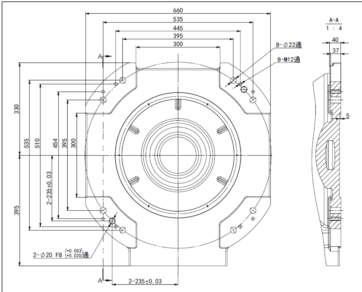
图 1.14 底座安装尺寸 (ER100B-3500-DW)
