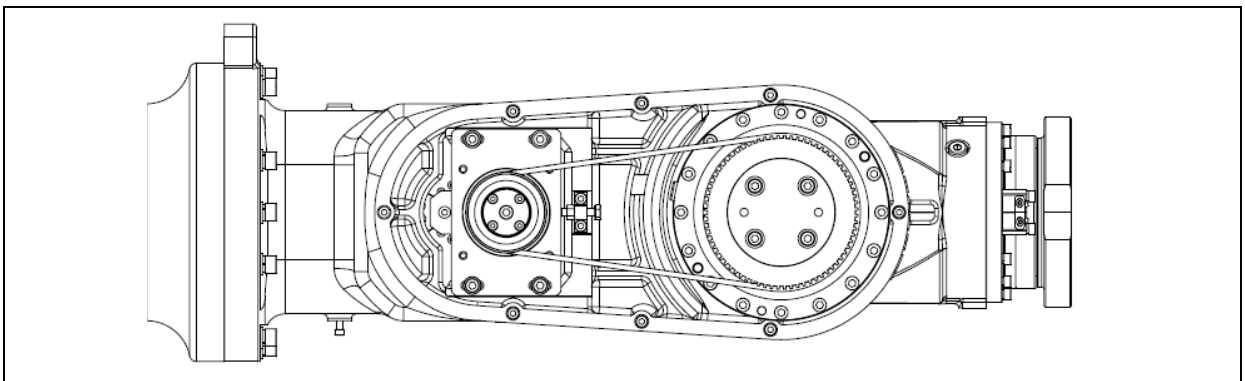
图 5.5 同步带张紧位置示意图 (ER100B-3000, ER100B-3500-DW)
