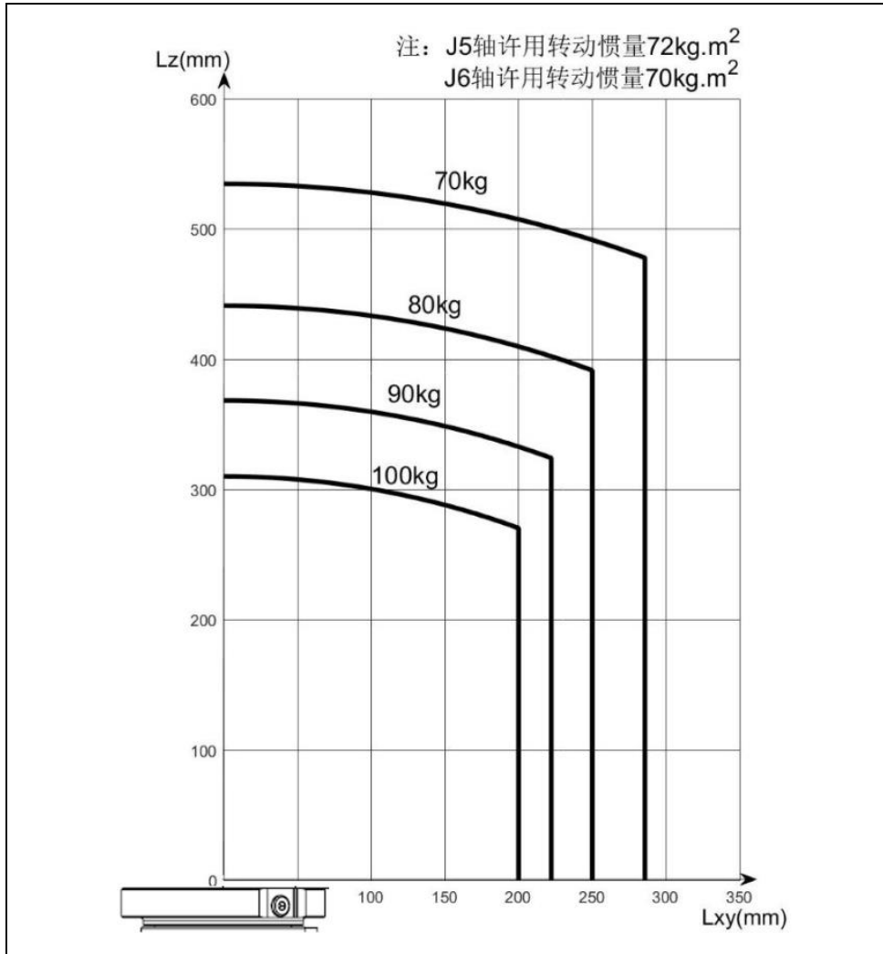
图 3.18 手腕部负载条件 (ER100B-3000, ER100B-3500-DW)
