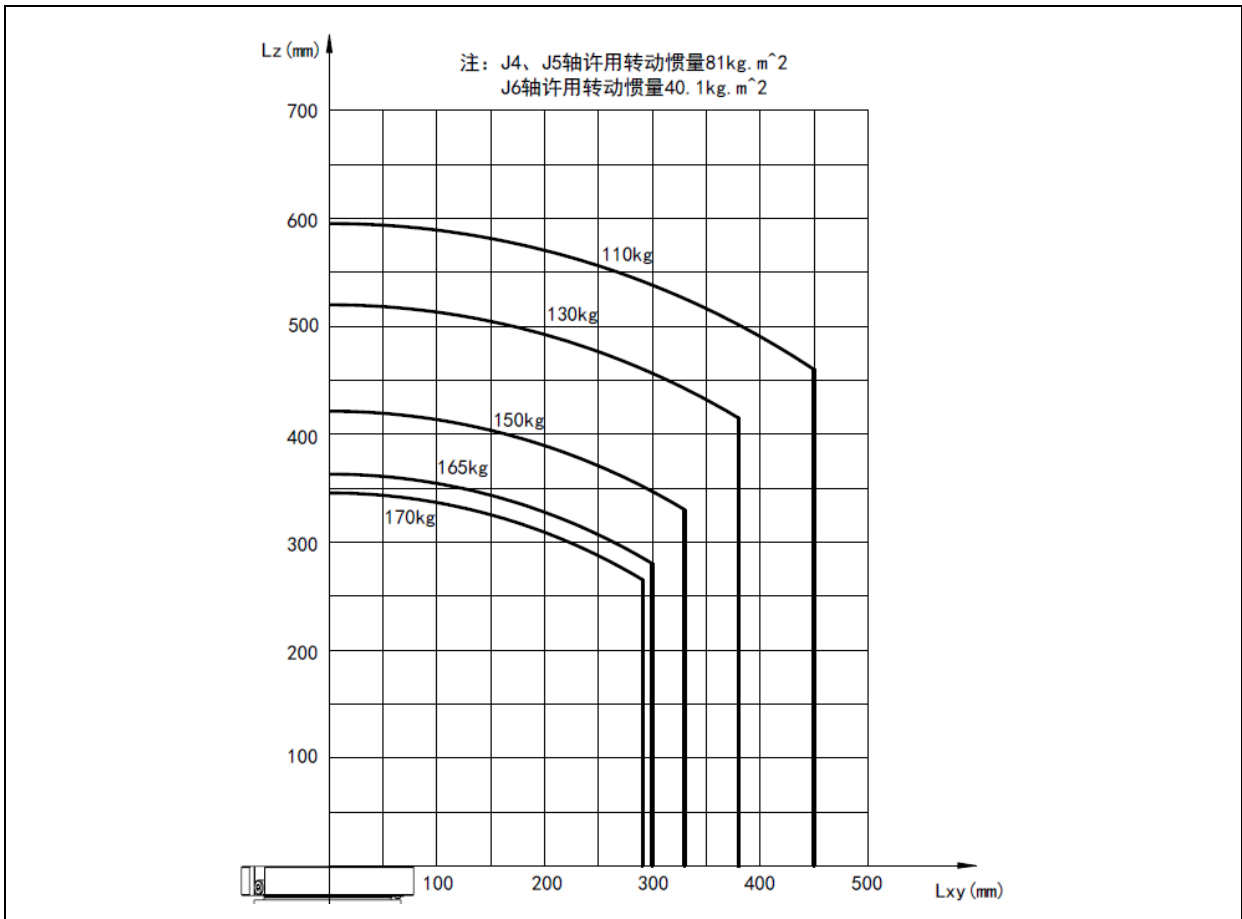
图 3.20 手腕部负载条件 (ER170B-2650)
