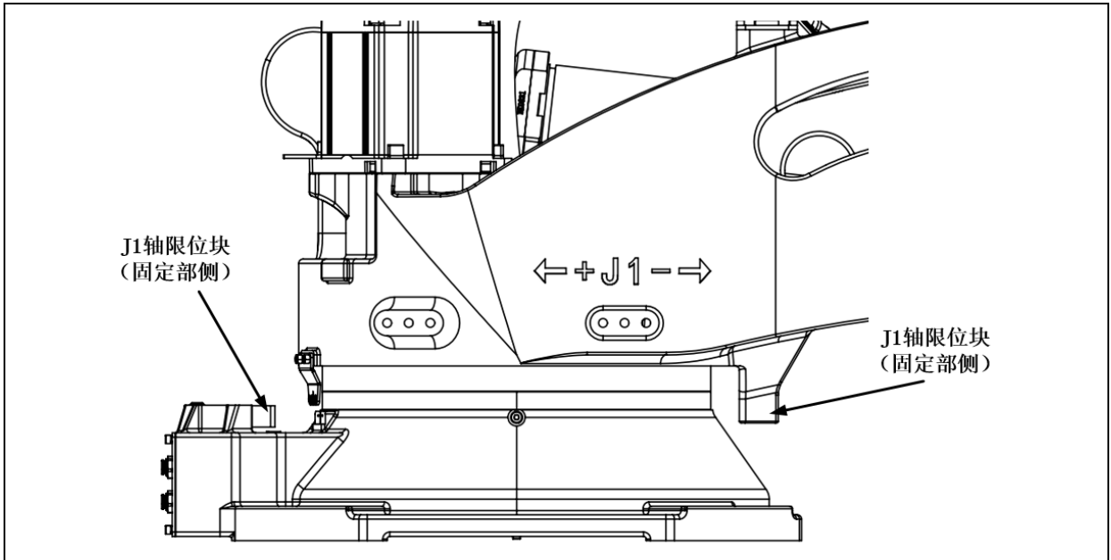
图 3.12 J1 轴机械式制动器位置 (ER100B-3500-DW)
