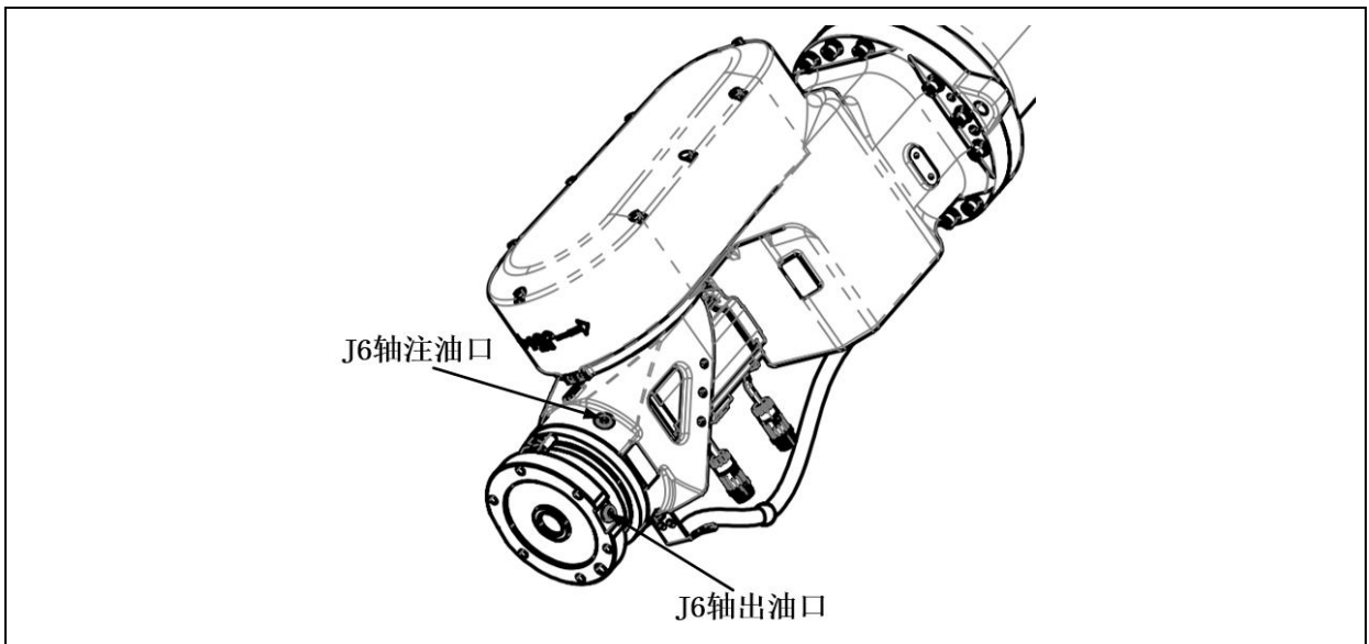
图 5.17 J6 轴注油、出油口 (ER100B-3000, ER100B-3500-DW, ER130B-3200)
