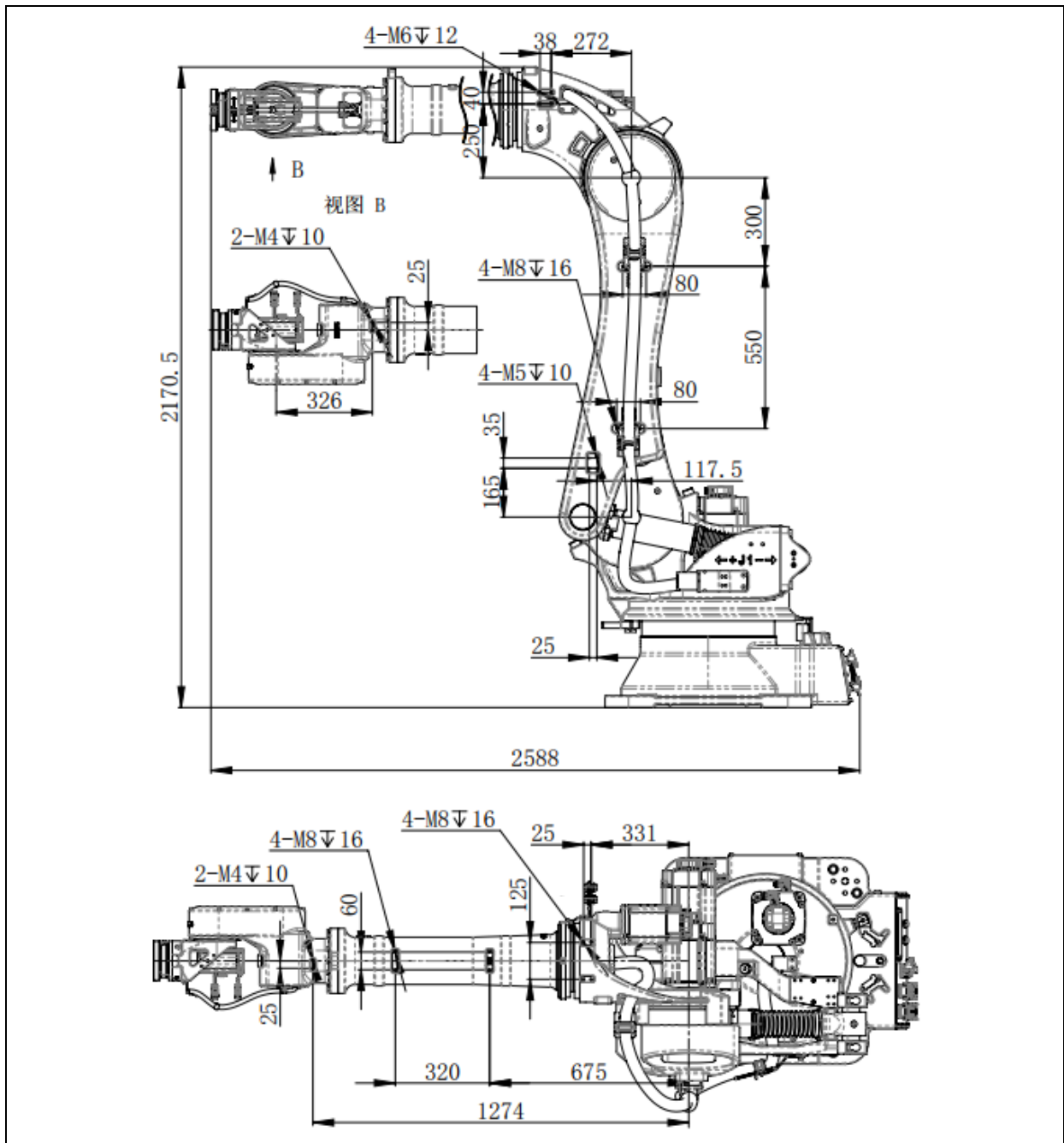
图 4.5 设备安装面尺寸 (ER100B-3000)
