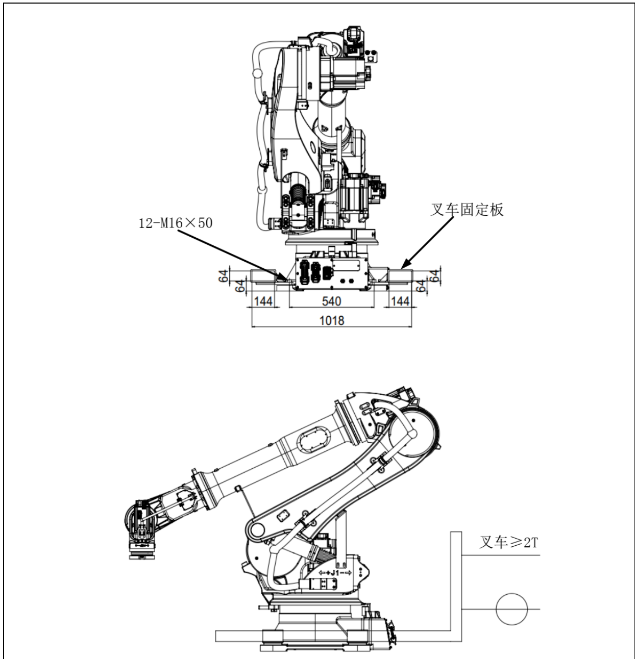
图 1.7 机器人叉车搬运示意图 (ER100B-3000,ER130B-3200,ER170B-2650,ER220B-2650)
