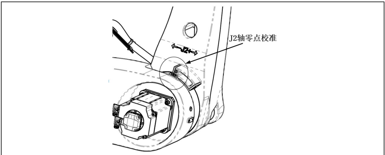
图 6.6 J2 轴零点校准示意图 (ER100B-3500-DW)
