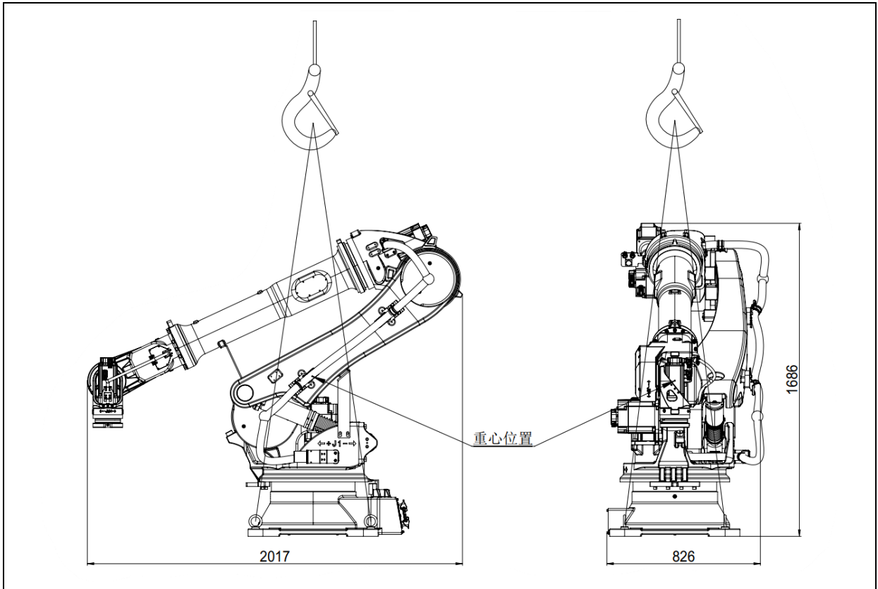
图 1.9 机器人起重机搬运示意图 (ER100B-3000, ER130B-3200, ER170B-2650, ER220B-2650)
