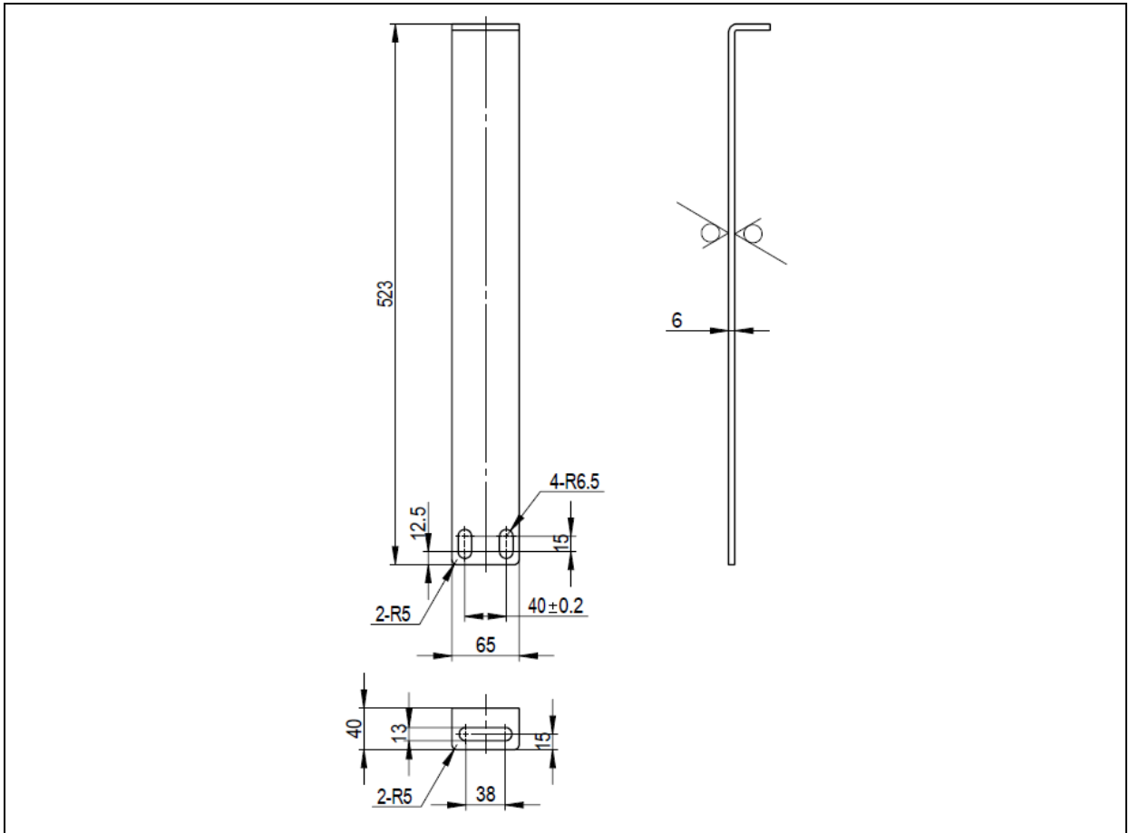
图 1.5 机器人固定支架示意图 5 (ER100B-3500-DW)
