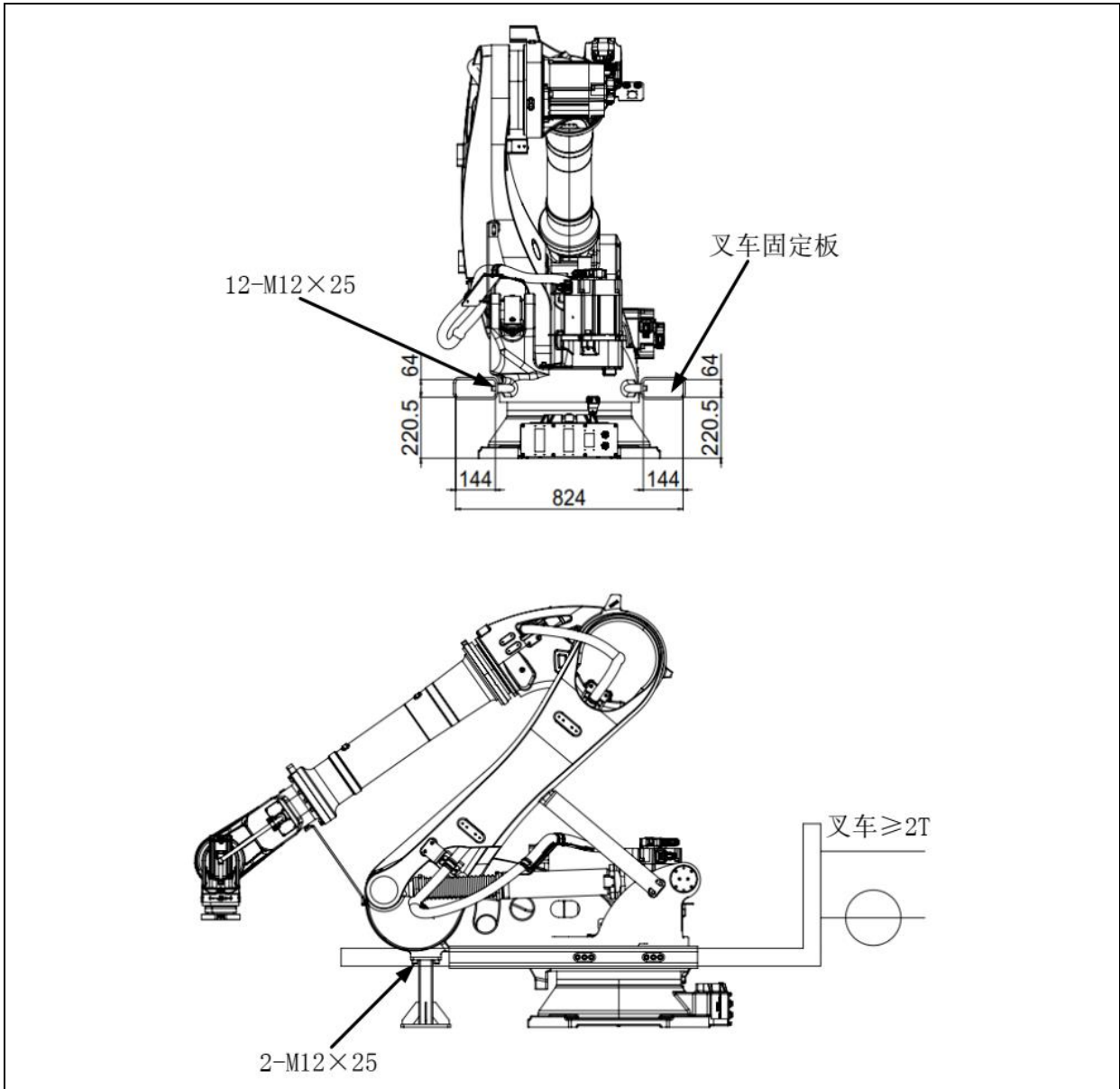
图 1.8 机器人叉车搬运示意图 (ER100B-3500-DW)
