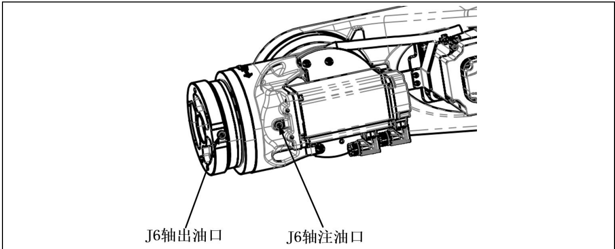
图 5.18 J6 轴注油、出油口 (ER170B-2650, ER220B-2650)
