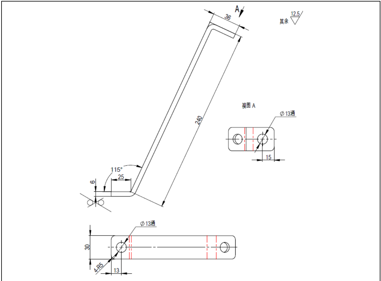
图 1.3 机器人固定支架示意图 3 (ER130B-3200)
