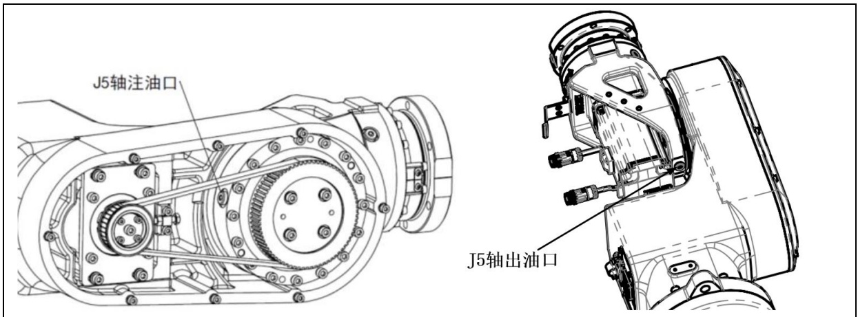
图 5.16 J5 轴注油、出油口 (ER100B-3500-DW)
