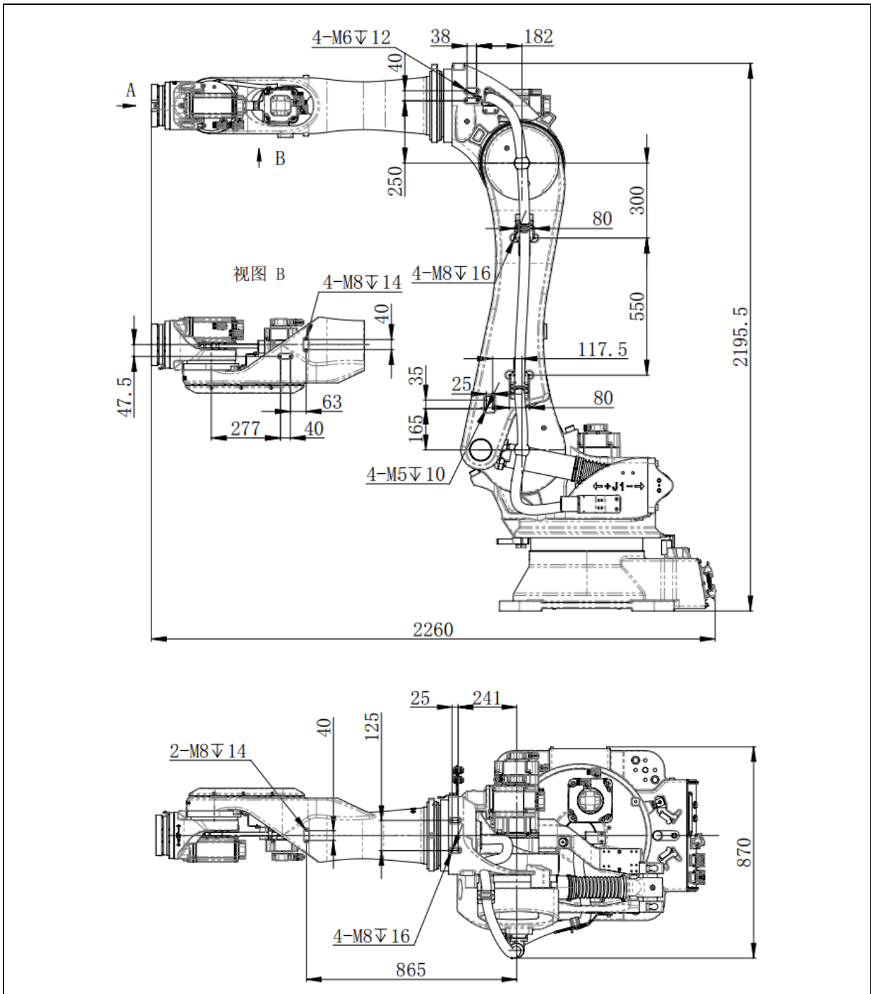
图 4.9 设备安装面尺寸 (ER220B-2650)
