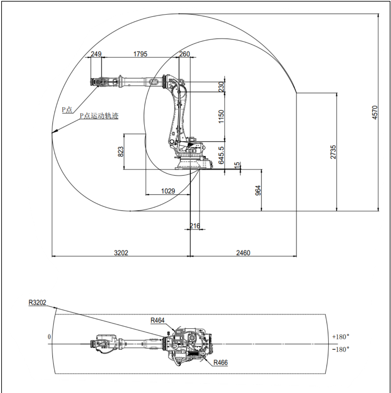
图 3.7 动作范围图 (ER130B-3200)
