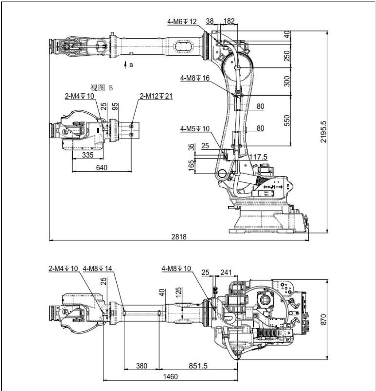
图 4.7 设备安装面尺寸 (ER130B-3200)
