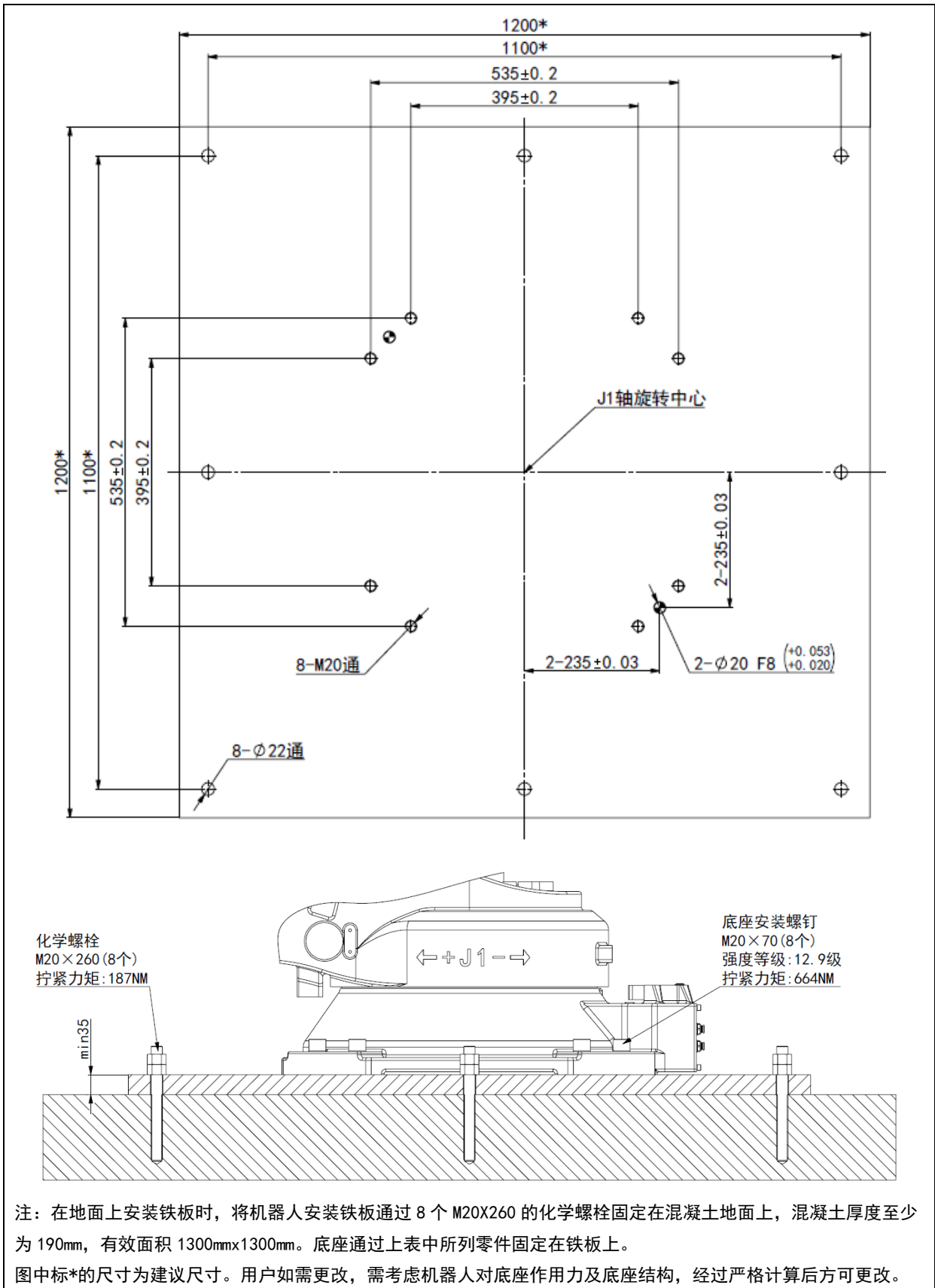
图 1.16 机器人安装铁板尺寸 (ER100B-3500-DW)
