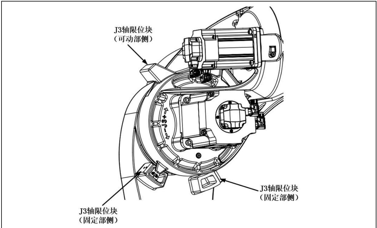
图 3.15 J3 轴机械式制动器位置
