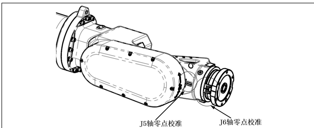
图 6.9 J5、J6 轴校准示意图 (ER100B-3000, ER100B-3500-DW, ER130B-3200)
