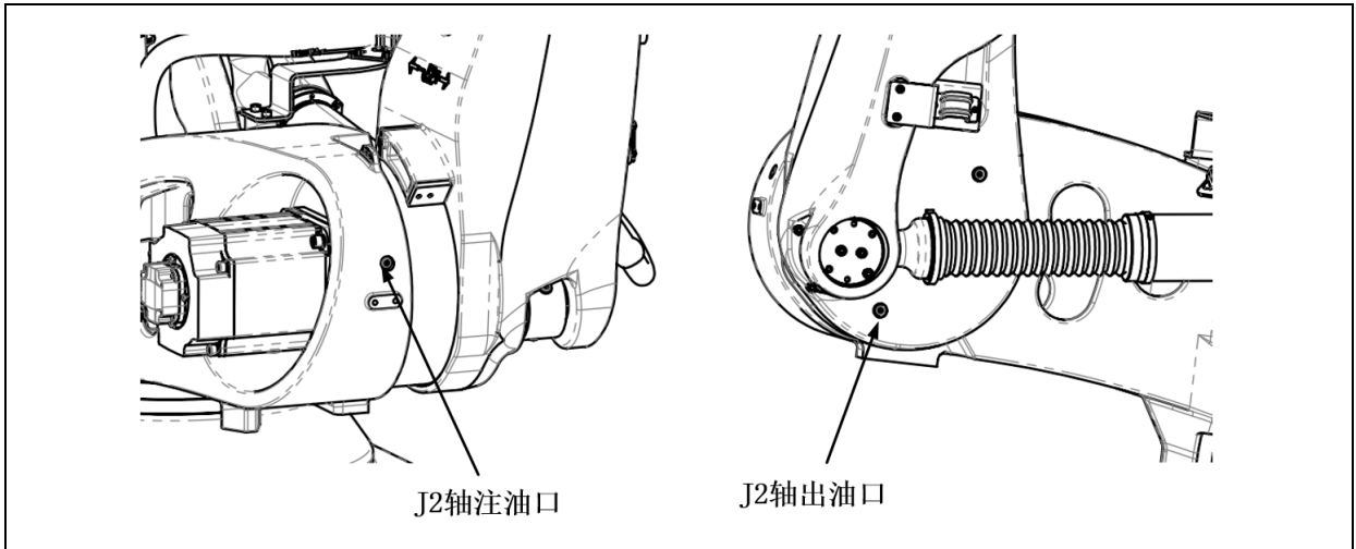
图 5.12 J2 轴注油、出油口 (ER100B-3500-DW)
