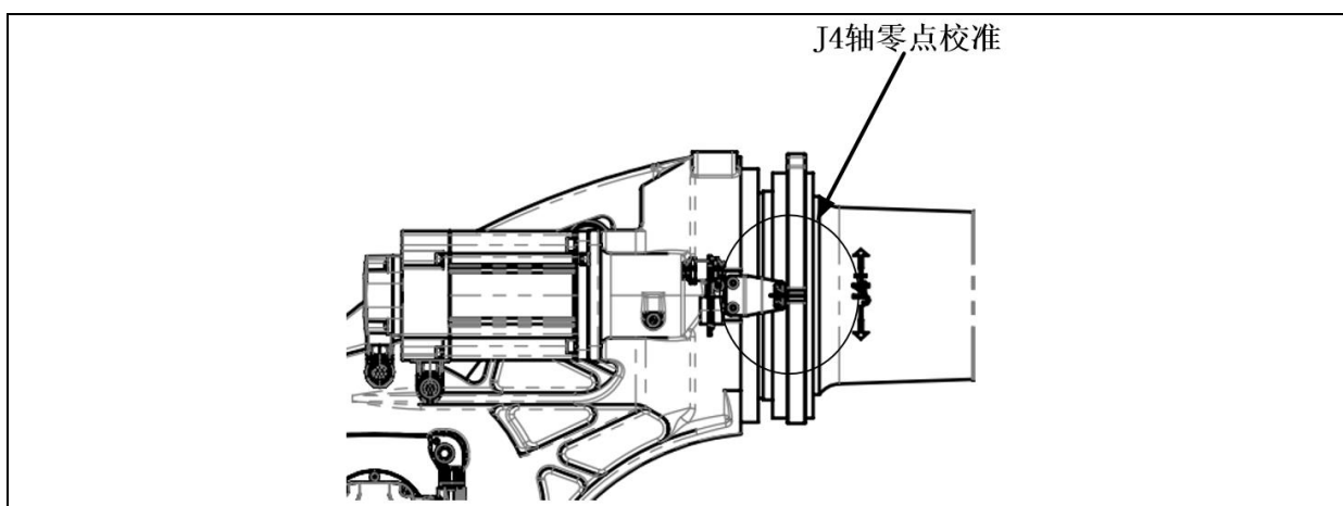
图 6.8 J4 轴校准示意图
