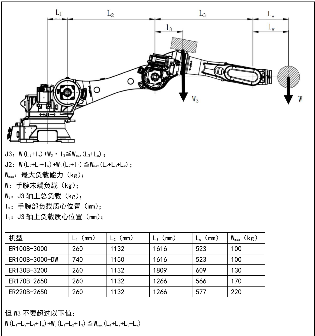
图 3.22 附加负载条件
