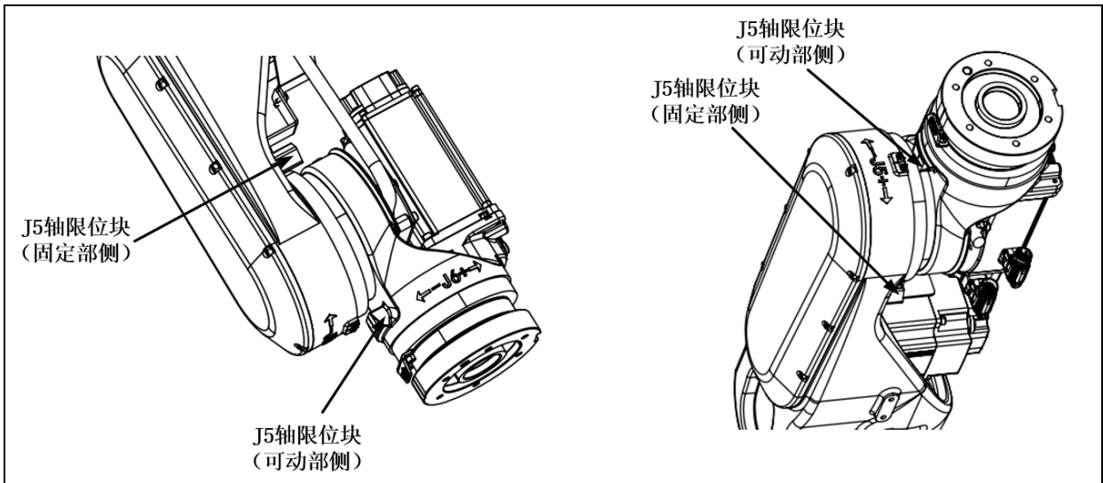
图 3.17 J5 轴机械式制动器位置 (ER170B-2650, ER220B-2650)
