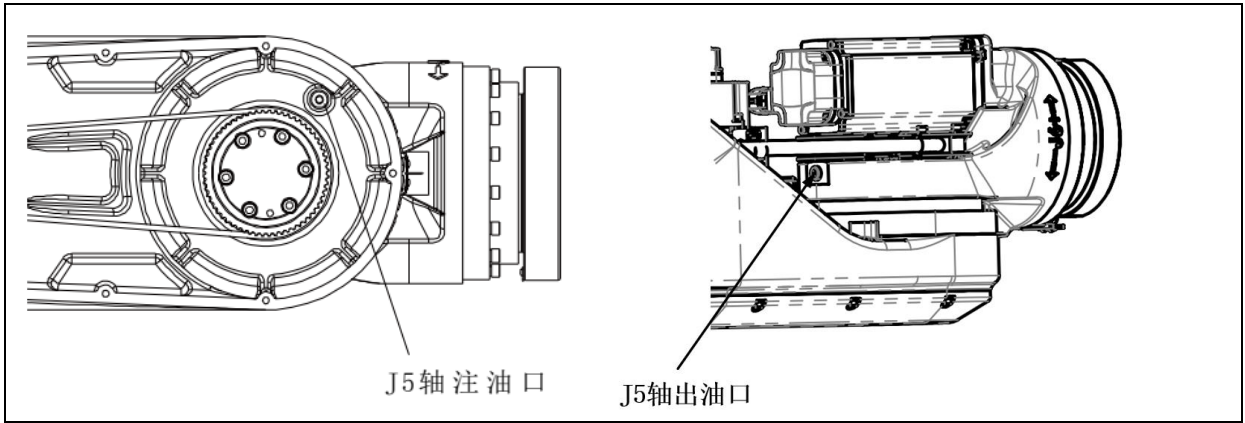
图 5.15 J5 轴注油、出油口 (ER100B-3000, ER130B-3200, ER170B-2650, ER220B-2650)
