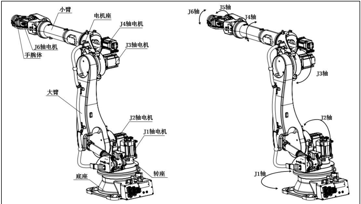
图 3.3 机器人的构成 (ER130B-3200)
