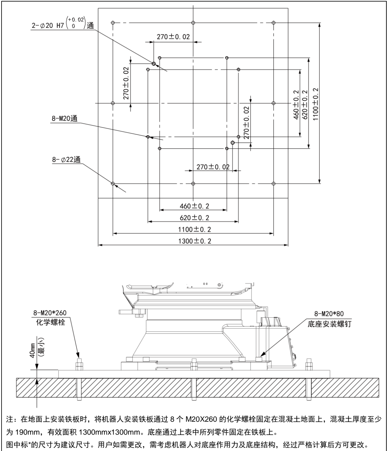
图 1.15 机器人安装铁板尺寸 (ER100B-3000, ER130B-3200, ER170B-2650, ER220B-2650)
