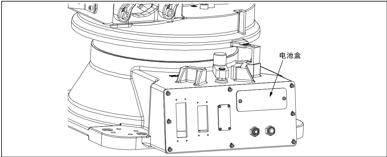
图 5.8 电池位置示意图
