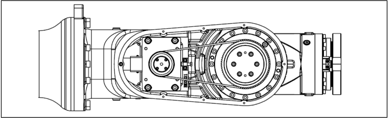
图 5.6 同步带张紧位置示意图 (ER130B-3200)
