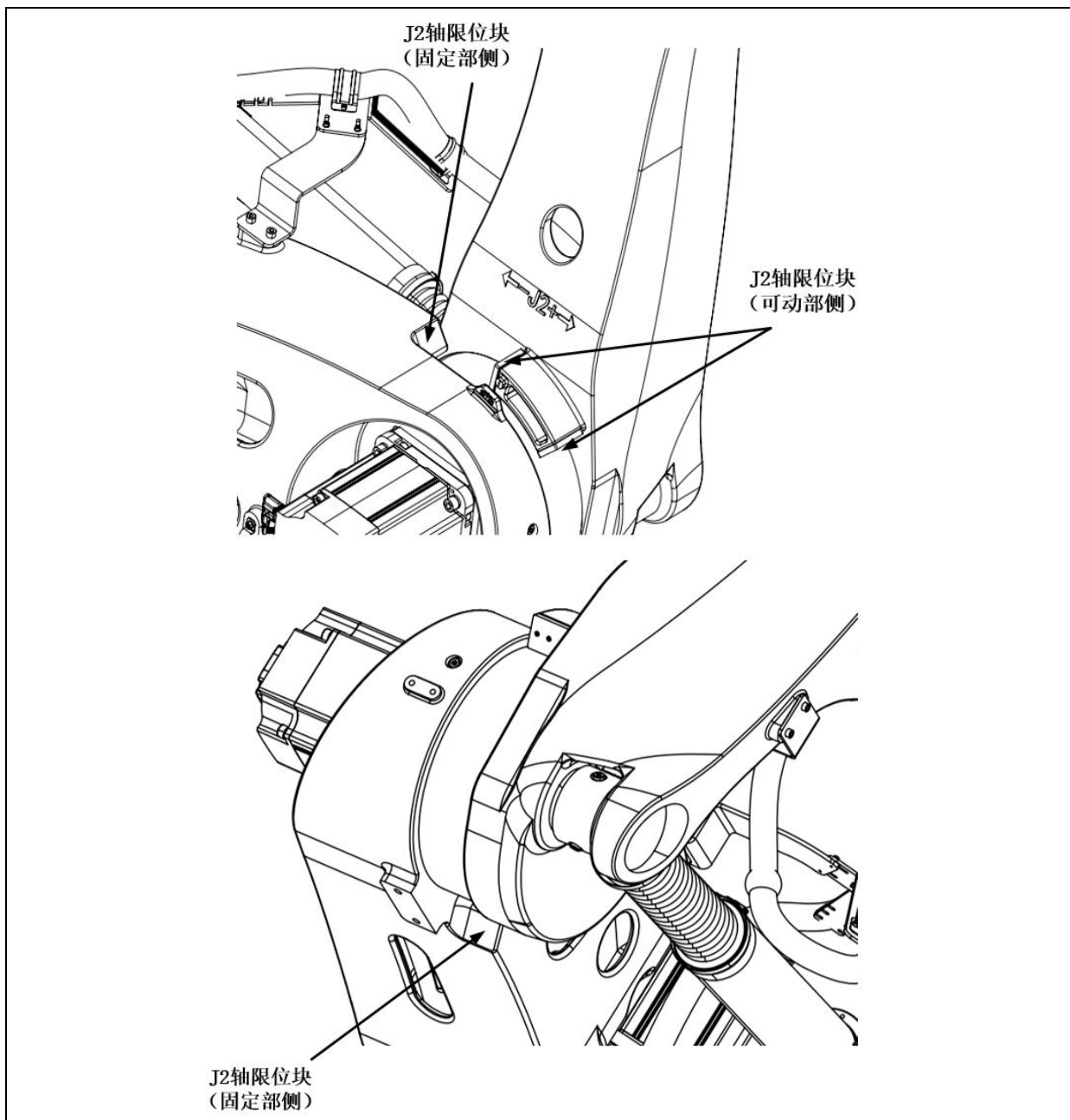
图 3.14 J2 轴机械式制动器位置 (ER100B-3500-DW)
