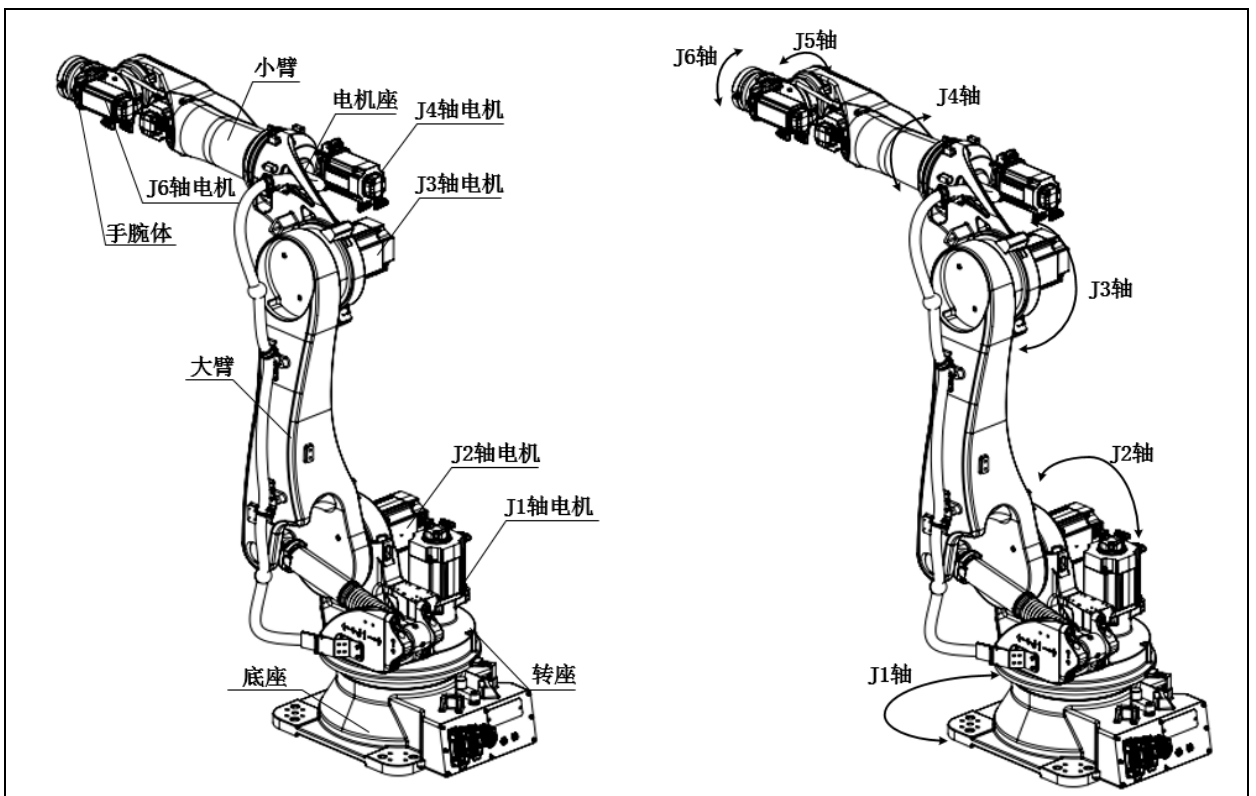
图 3.4 机器人的构成 (ER170B-2650, ER220B-2650)
