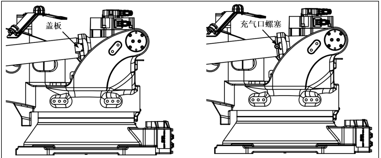
图 5.3 气弹簧检查示意图 (ER100B-3500-DW)
