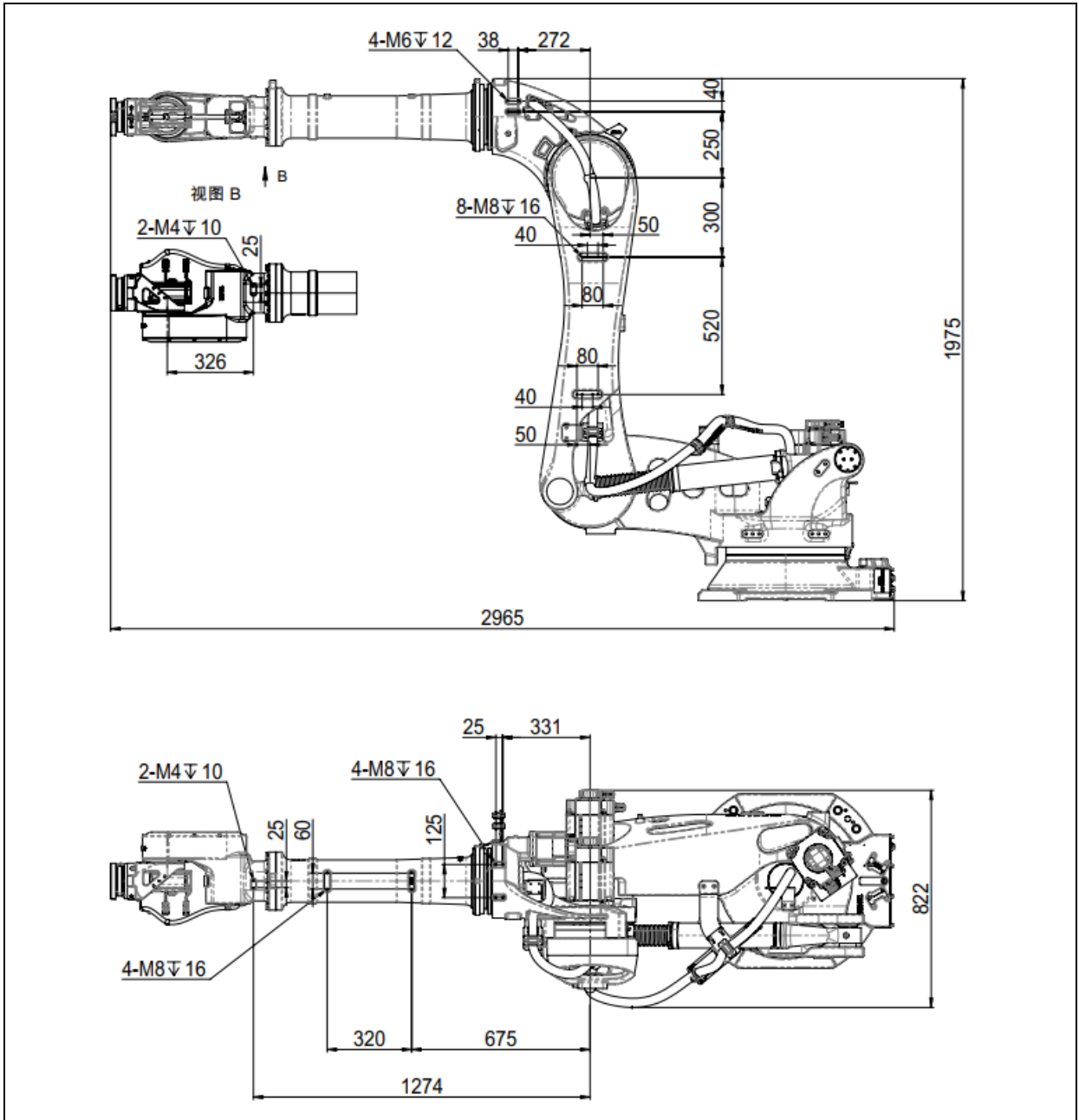
图 4.6 设备安装面尺寸 (ER100B-3500-DW)
