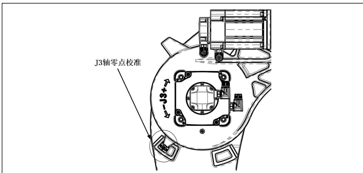
图 6.7 J3 轴校准示意图
