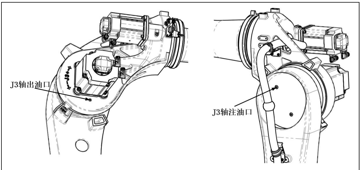
图 5.13 J3 轴注油、出油口
