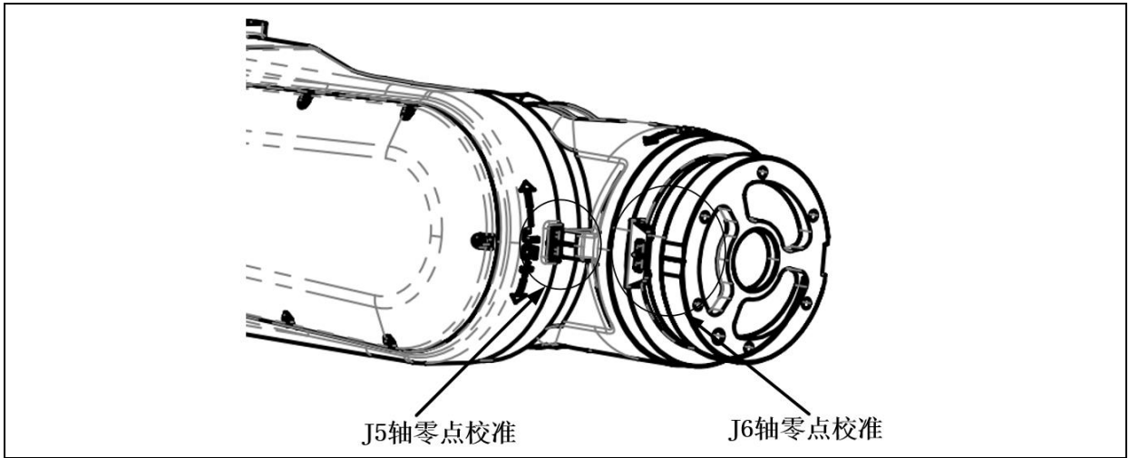
图 6.10 J5、J6 轴校准示意图 (ER170B-2650, ER220B-2650)
