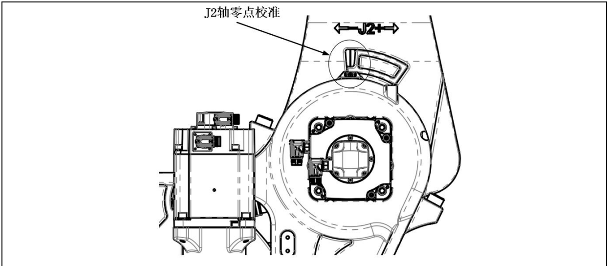
图 6.5 J2 轴校准示意图 (ER100B-3000, ER130B-3200, ER170B-2650, ER220B-2650)
