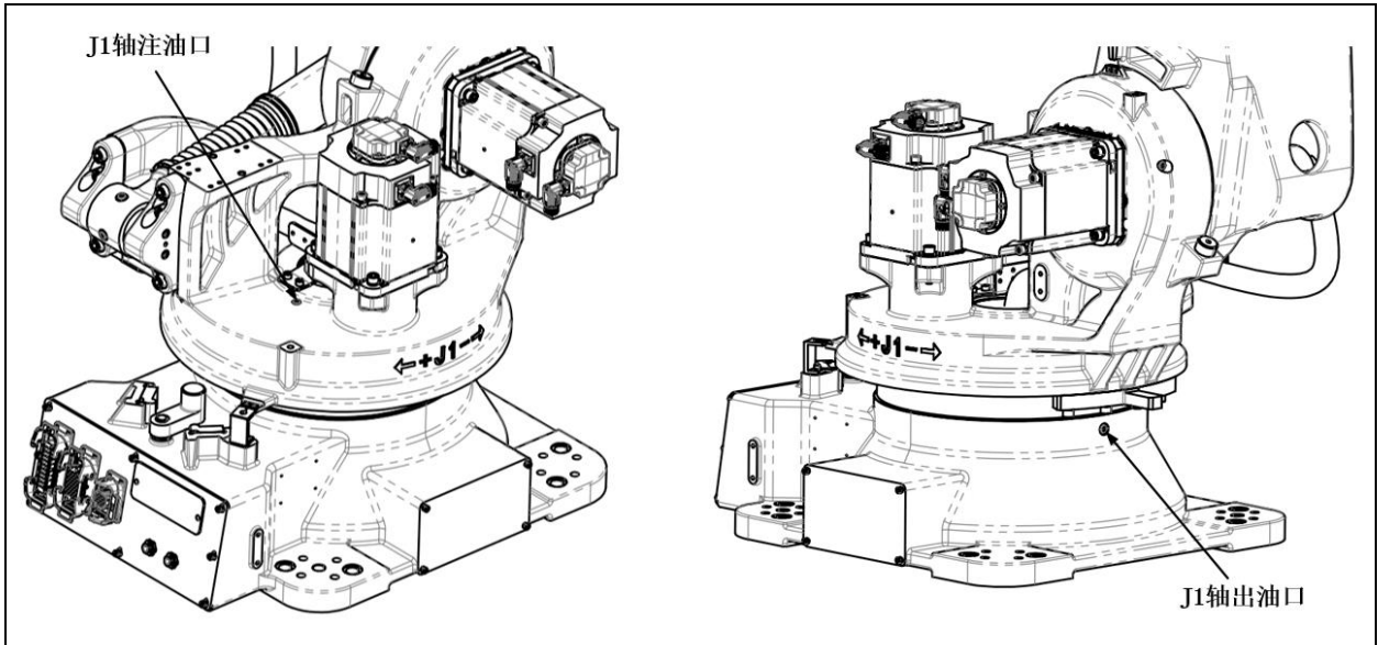
图 5.9 J1 轴注油、出油口 (ER100B-3000, ER130B-3200, ER170B-2650, ER220B-2650)
