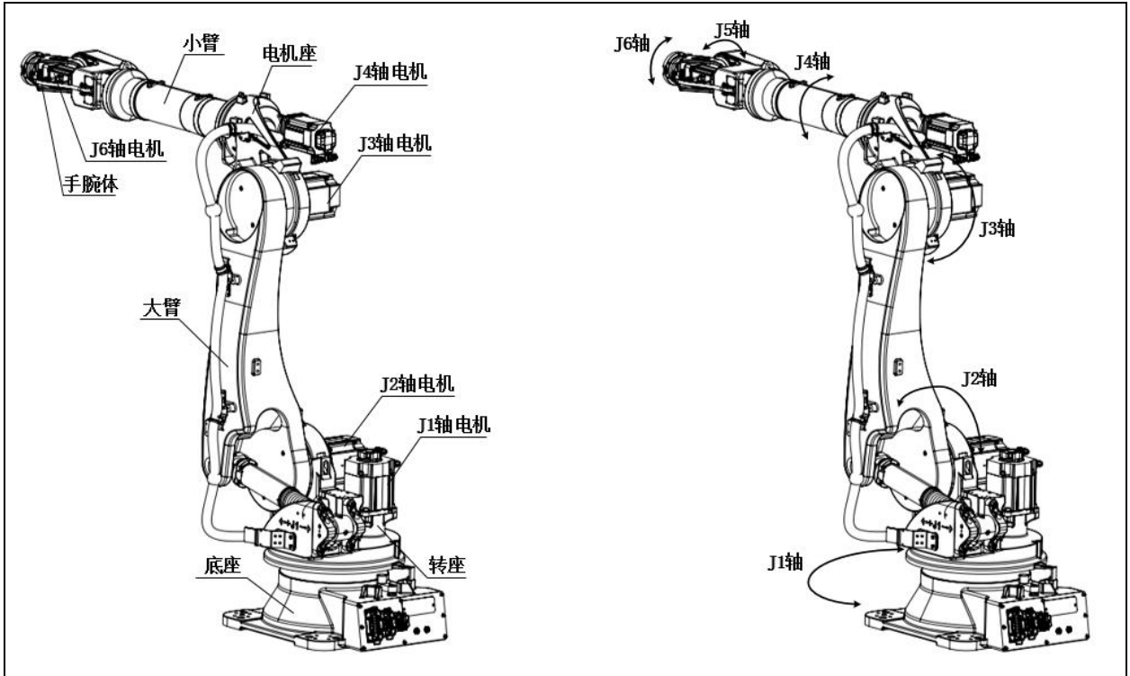
图 3.1 机器人的构成 (ER100B-3000)
