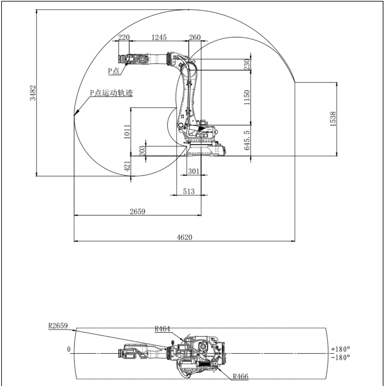
图 3.8 动作范围图 (ER170B-2650)
