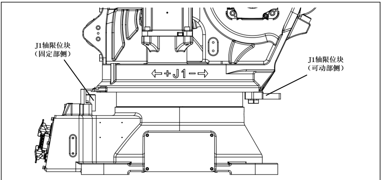
图 3.11 J1 轴机械式制动器位置 (ER100B-3000, ER130B-3200, ER170B-2650, ER220B-2650)
