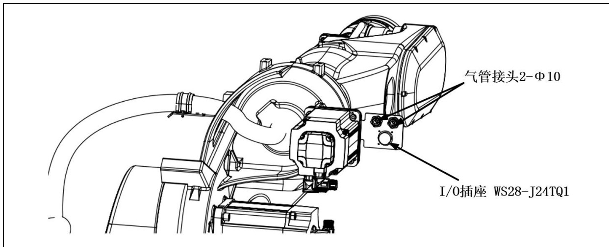
图 4.10 外部管线示意图
