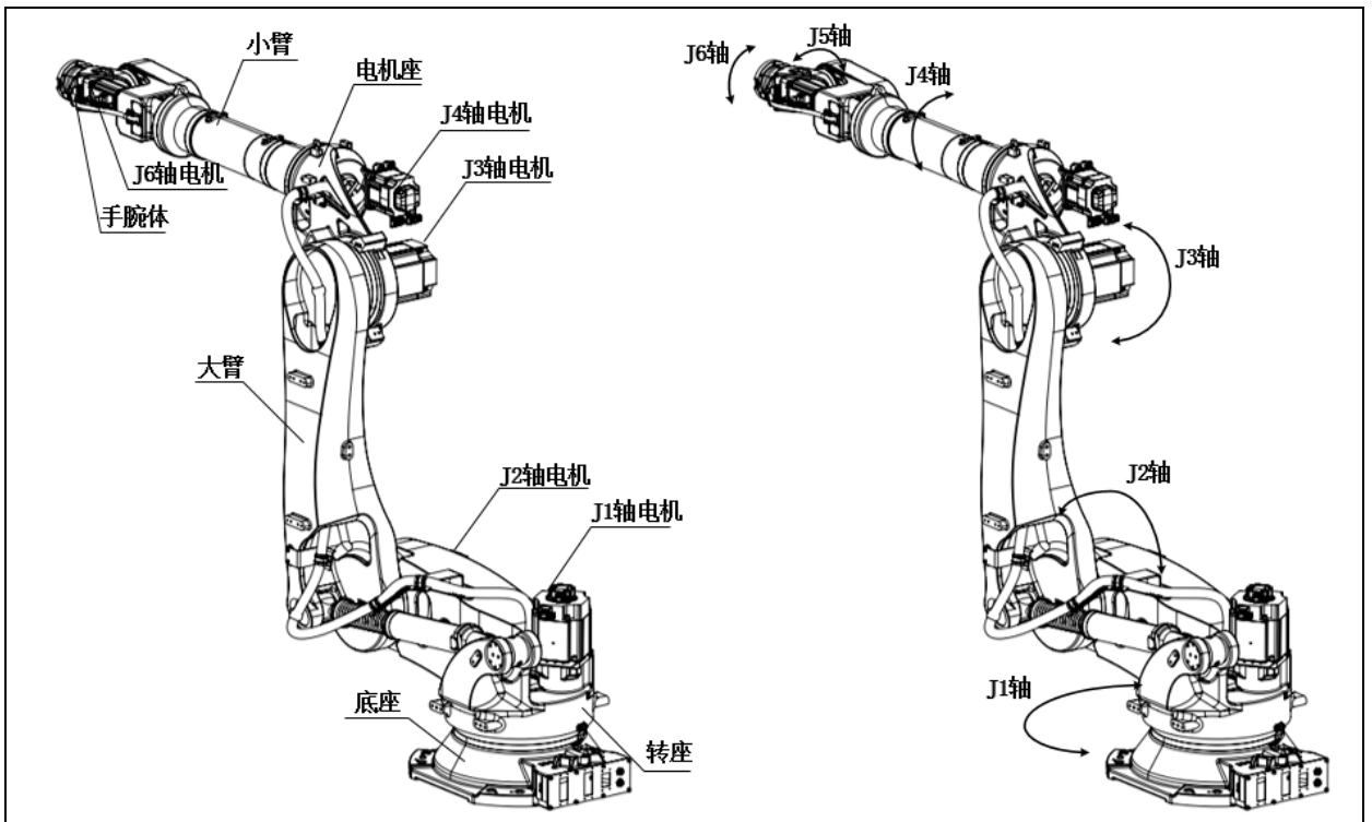
图 3.2 机器人的构成 (ER100B-3500-DW)
