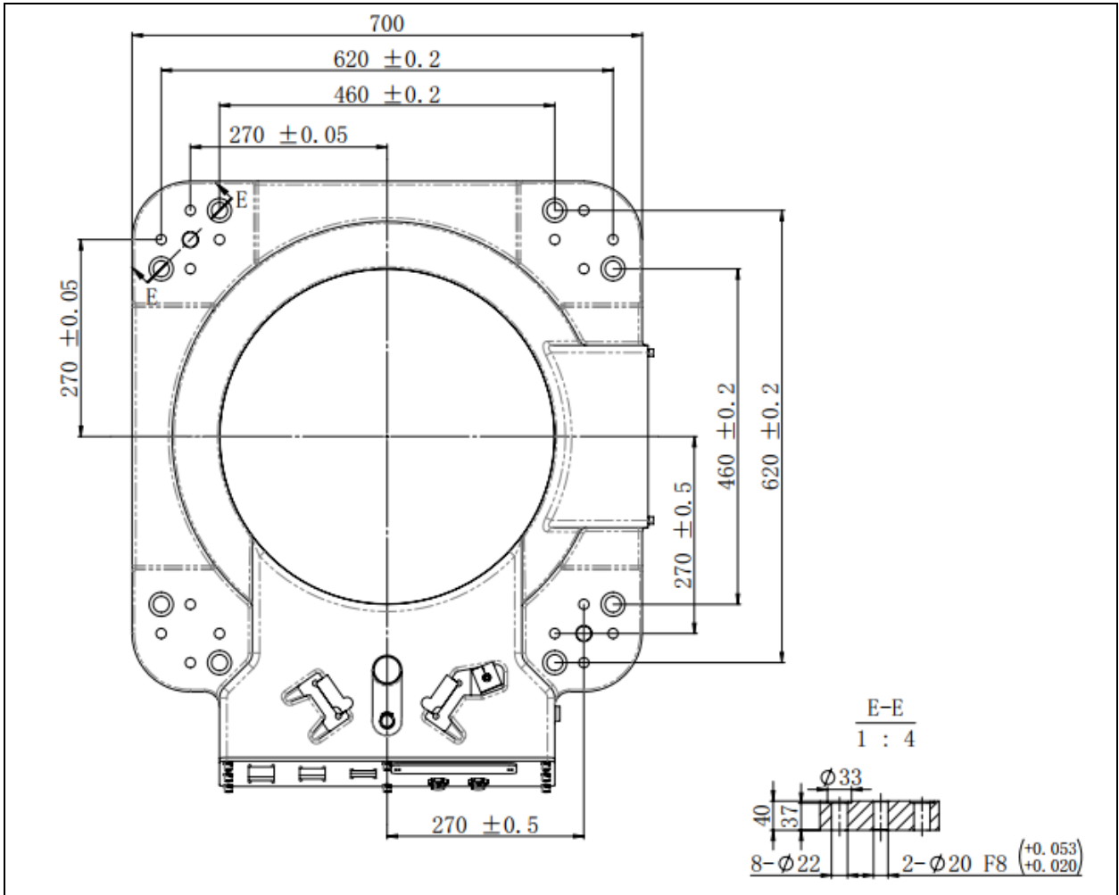
图 1.13 底座安装尺寸 (ER100B-3000, ER130B-3200, ER170B-2650, ER220B-2650)
