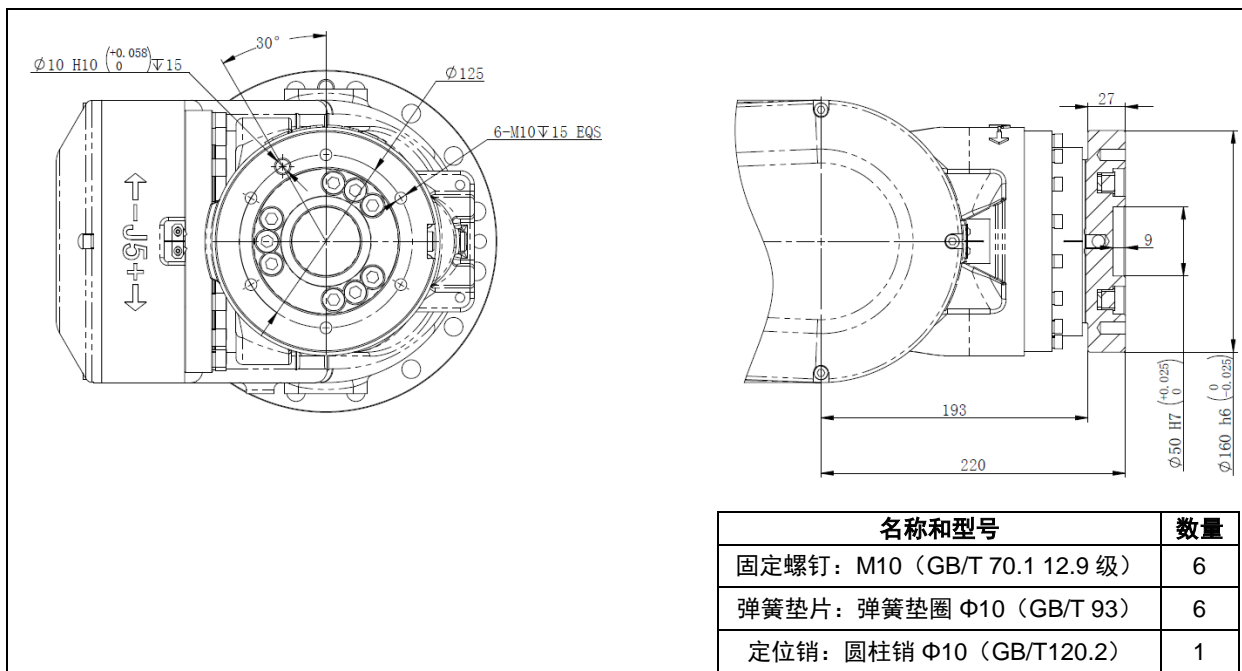
图 4.3 末端法兰安装接口 (ER170B-2650)
