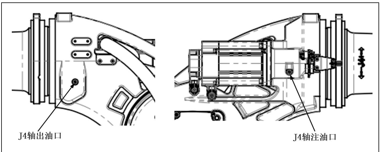
图 5.14 J4 轴注油、出油口
