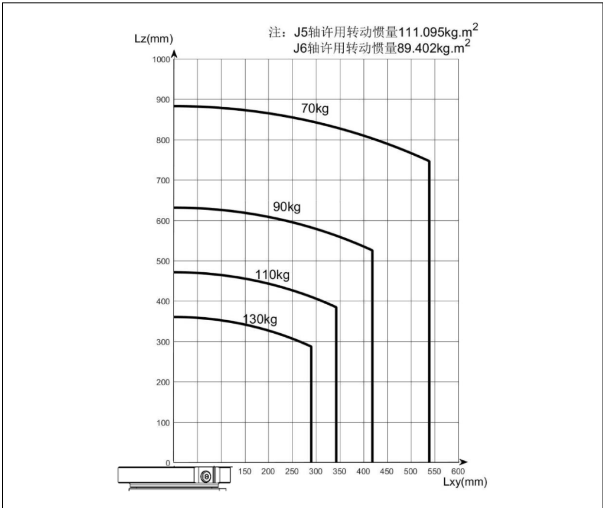
图 3.19 手腕部负载条件 (ER130B-3200)
