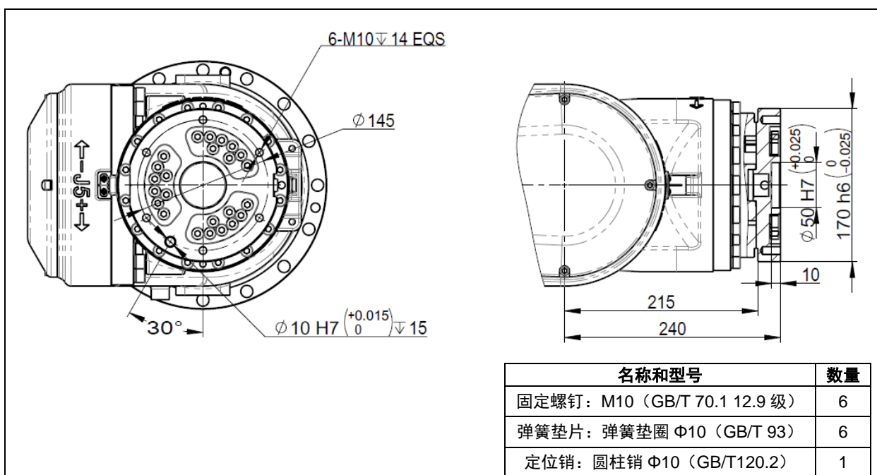
图 4.4 末端法兰安装接口 (ER220B-2650)
